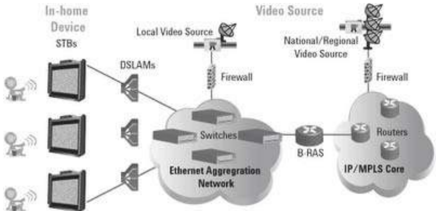
ตัวอย่าง Network Configuration ของโทรทัศน์ไอพี (IPTV)
