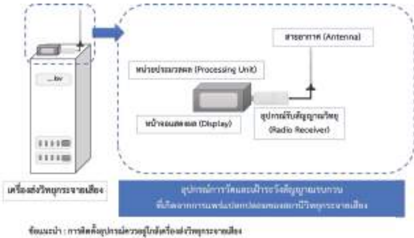
รูปที่ 1 การติดตั้งอุปกรณ์การวัดและเฝ้าระวังสัญญาณรบกวนที่เกิดจากการแพร่ปลอมของสถานีวิทยุกระจายเสียง
