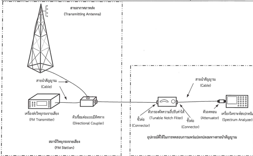
รูปที่ 1 แผนผังการต่อเครื่องมือสำหรับการทดสอบการแพร่ปลอมผ่านสายนำสัญญาณ
