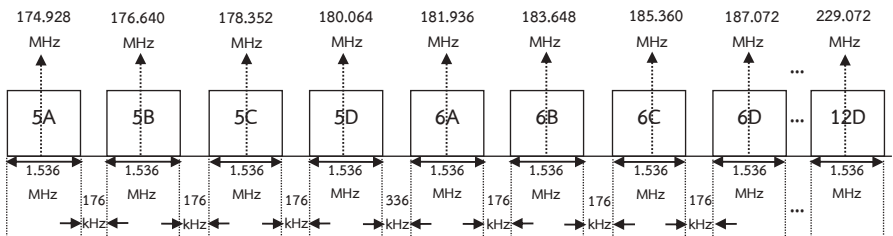
รูปที่ 1 แผนภาพบล็อกความถี่วิทยุ ความถี่วิทยุที่กึ่งกลาง ความกว้างแถบคลื่นความถี่ และความกว้างแถบคลื่นความถี่ป้องกัน
