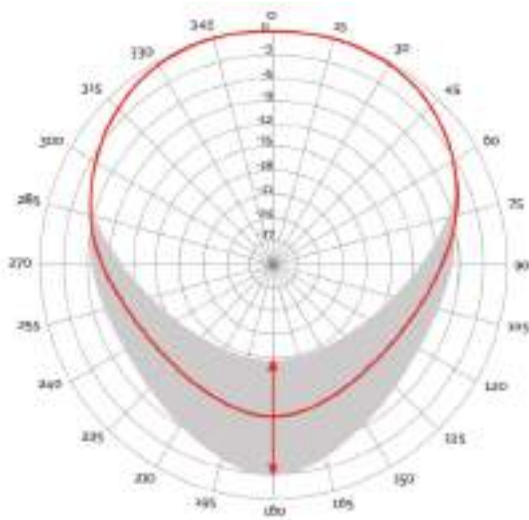
รูปที่ 1 แสดงแบบรูปกำลังของสายอากาศรับสัญญาณภายในอาคารแบบแอกทีฟ แบบที่ 1
