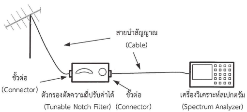
สายอากาศภาครับ (Receiving Antenna)
